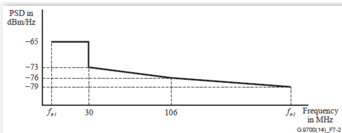
Slika 4.9.2 - Maska PSD za G.fast 212 MHz profil*
