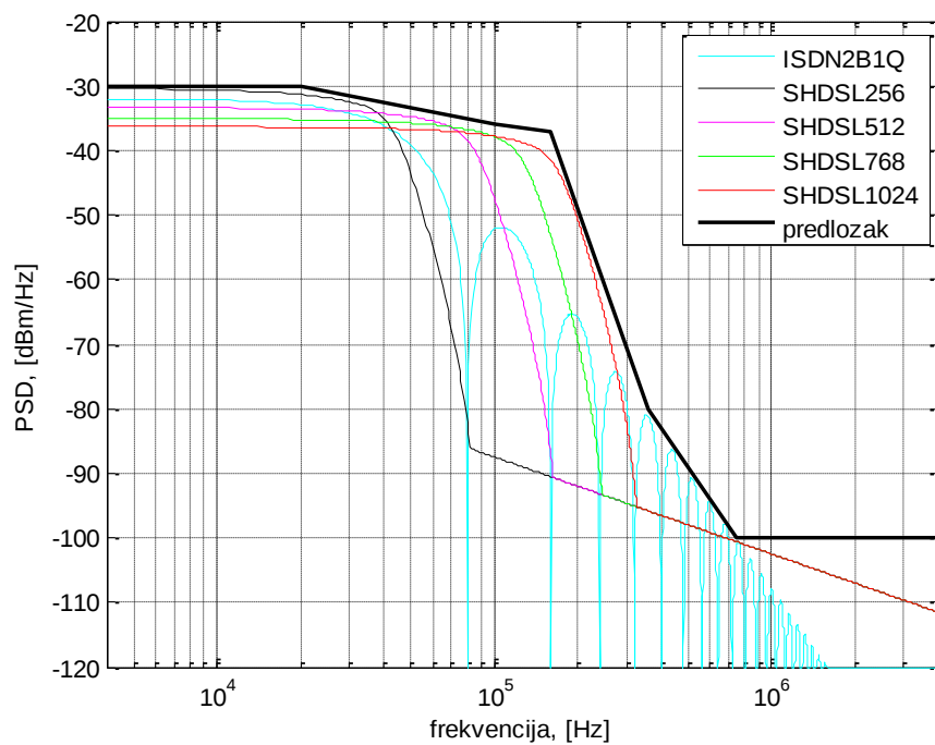
Slika 5.7.7 Frekvencijski predložak za odlazni smjer prijenosa (duge pretplatničke linije) za ADSL preko POTS (aneks A).
