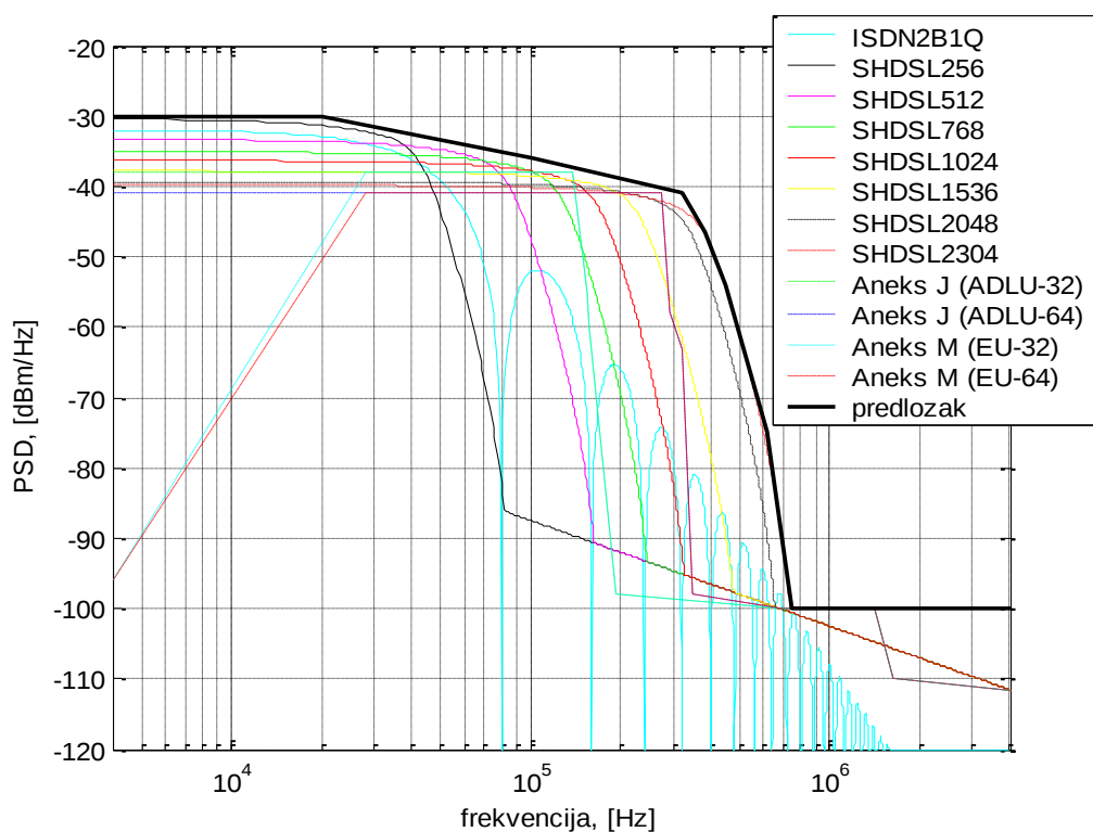
Slika 5.7.5 Frekvencijski predložak za odlazni smjer prijenosa (pretplatničke linije srednje duljine).
