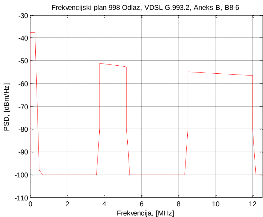
Slika 5.7.2 Frekvenzijski predložak za odlazni smjer prijenosa za VDSL2, frekvenzijski plan 998, B8-6
