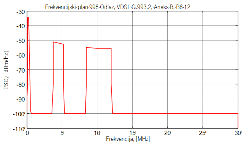
Slika 5.7.3 Frekvencijski predložak za odlazni smjer prijenosa za VDSL2, frekvencijski plan 998, B8-12
