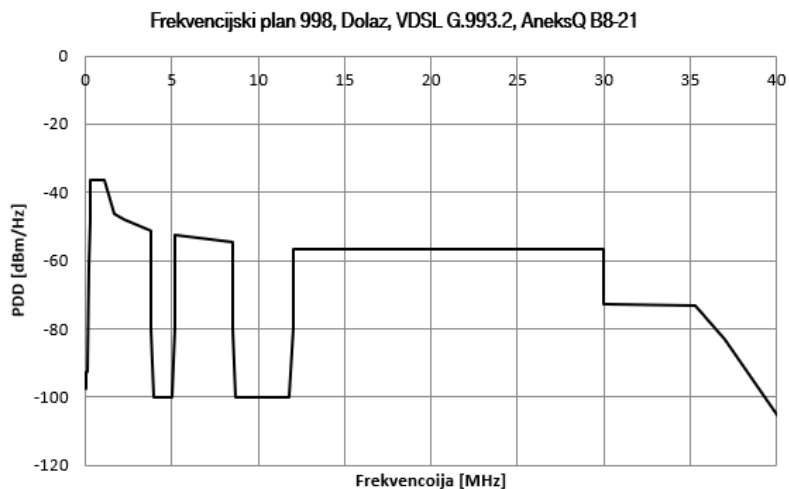
Slika 5.6.1 Frekvencijski predložak za VDSL2 frekvencijski plan 998, B8-21 dolaz (crno).
