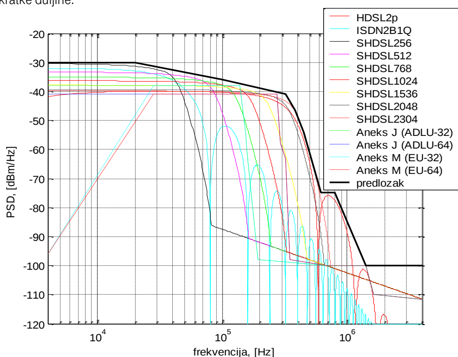
Slika 5.7.1 Frekvencijski predložak za odlazni smjer prijenosa (kratke pretplatničke linije).
