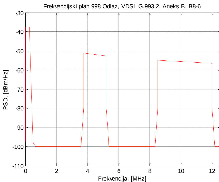
Slika 4.8.3 Maska PSD za VDSL2 frekvencijski plan 998, B8-6 odlaz (crveno) Slikama 4.8.4. i 4.8.5. dane su maske PSD za VDSL2 frekvencijski plan 998, B8-12 dolaz (sl. 4.8.4) i odlaz (sl. 4.8.5)
