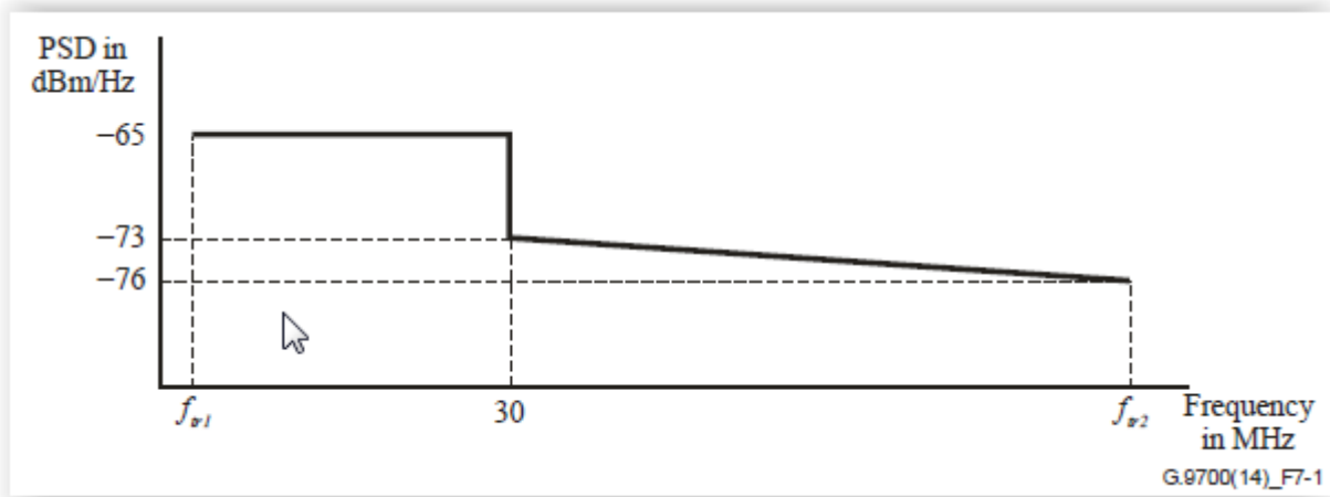
Slika 4.9.1 - Maska PSD za G.fast 106 MHz profil
