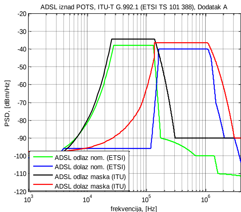
Slika 4.4.1. Maske i nominalne maske spektralne gustoće snage za ADSL iznad POTS-a.
