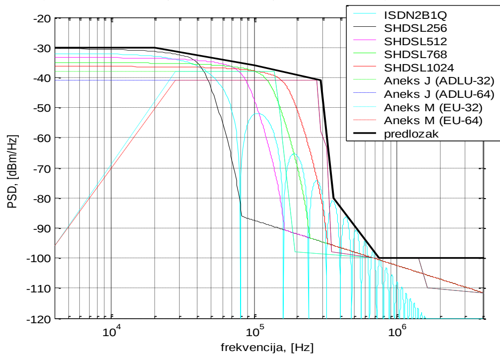
Slika 5.7.6 Frekvencijski predložak za odlazni smjer prijenosa (duge pretplatničke linije) za ADSL preko ISDN (aneks B).
